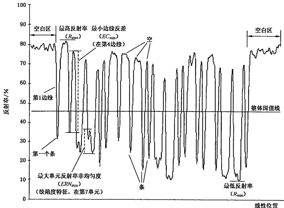
图 2 扫描反射率曲线特征示意图
